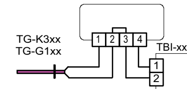
Abb 6: Ext., seperater Fühler bei Verwendung von einem TBI-xx als ext. Sollwertpotentiometer
