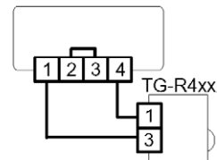
Abb 3: Raumfühler TG-R430 bei ext. Sollwert und Fühler
