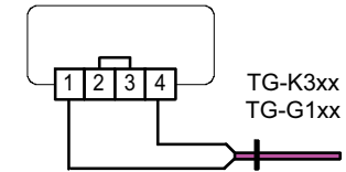
Fig 4: Boden- oder Kanalfühler bei int. Sollwert
