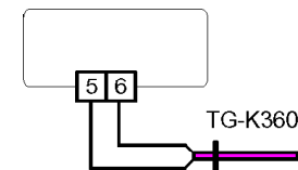
Abb 7: Begrenzungsfühler
