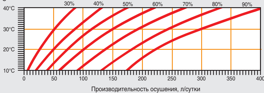
Температура воздуха, °C DH 300 Y
