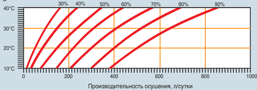
Температура воздуха, °C DH 600 Y
